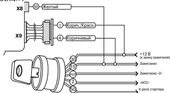
Типовая схема подключения к замку зажигания (параллельно)
