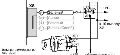
Пример схемы блокировки нормально разомкнутым реле (перепрограммировать тип контактов НР) Рис. 12
