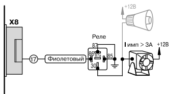
Схема подключения сирены или группы сирен с суммарным током потребления более 3А Рис. 13
