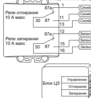
Схема подключения к блоку ЦЗ с управлением импульсами положительной полярности в водительской двери
